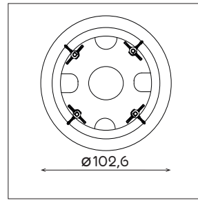
Bild 3: Baldachin (Vorderansicht)
