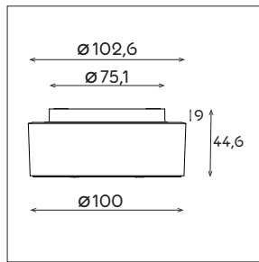
Bild 2: Baldachin (Seitenansicht)
