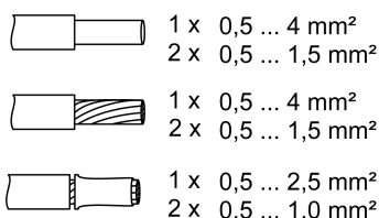
Bild 3: Klemmbare Leiterquerschnitte
