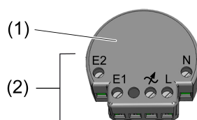
Bild 1: Geräteaufbau
